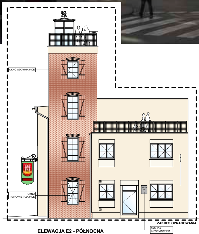
ELEWACJA E2 - PÓŁNOCNA
