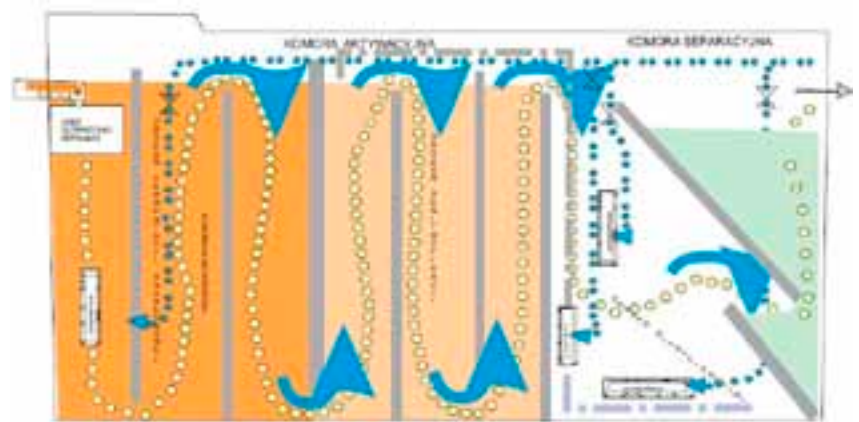
Schemat kompaktu biologicznego oczyszczania - osad czynny, metoda przepływowa
